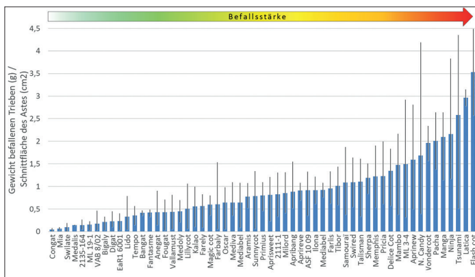
Abb. 7: Stark unterschiedliche Sortenanfälligkeit gegenüber Monilia in Sortenversuchen im Wallis im Durchschnitt von drei Jahren (2017, 2018 und 2019). Die schwarzen Linien zeigen die maximale und minimale Befallsstärke in den drei Erhebungsjahren. Die Befallsstärke wurde mit Methode der Gewichtsbestimmung der befallenen Astpartien pro Baum (g) im Vergleich zur Schnittfläche des Astes (cm²) ermittelt.
