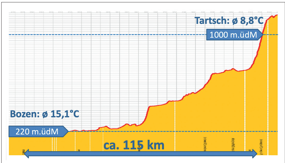
Abb. 8: Verschiedene Höhenstufen mit unterschiedlichen klimatischen Bedingungen
